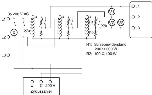
Anschlussplan 2
